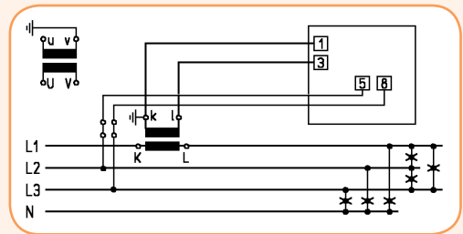
Схема подключения счетчика WS 1202
