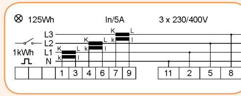
Схема подключения счетчика WS 1102
